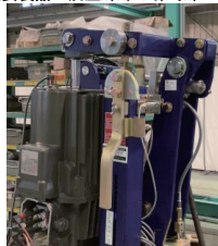
主要製品：油圧スラスタ式ディスクブレーキ
